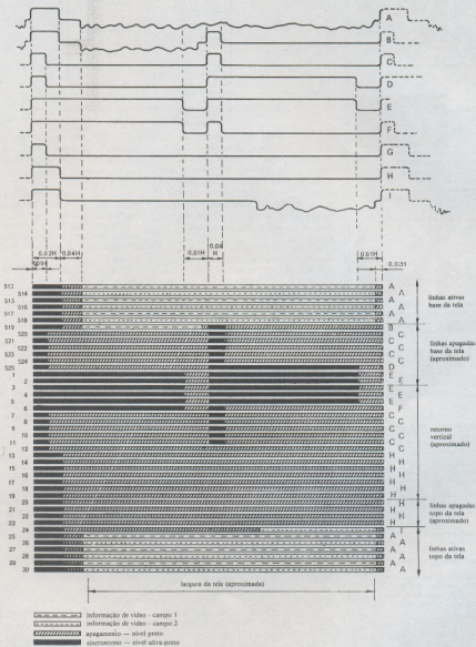
Fig. 14 - IV Detalhes do apagamento e sincronismo verticais (martelo de sincronismo).
