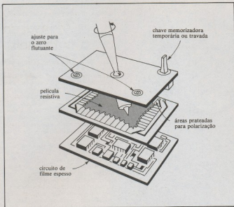
Um joystick sofisticado — Ao se movimentar a alavanca deste joystick, provoca-se alterações na polaridade da película resistiva, resultando em 2 tensões analógicas, proporcionadas à posição do contato.
