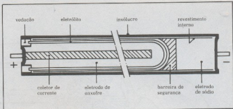
Vista em corte de uma bateria sódio-enxofre de 300 Wh.
