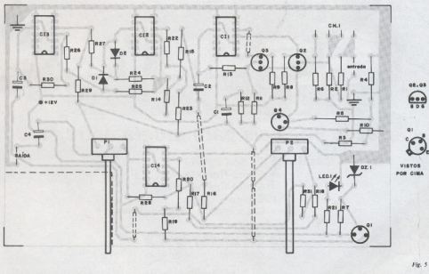
Placa de circuito impresso do alterador de formas de onda, vista pelo lado cobreado e também pelo dos componentes (em transparência). Ela está representada em seu tamanho natural de 15 por 10 cm, aproximadamente. No canto inferior esquerdo (face dos componentes) foi previsto um espaço para a eventual instalação de uma bateria.
