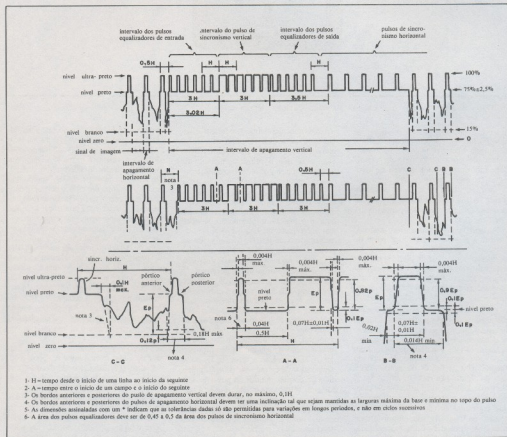
Fig. 12 - IV Forma de onda do sincronismo em TV (padrões FCC).
