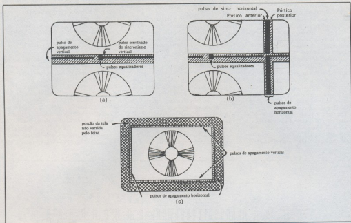
Fig. 13 - IV Dessincronização vertical e horizontal; redução de altura e largura na tela.
