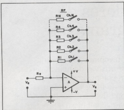
Fig. 3 A malha chaveada de entrada da figura 2 poderá ser trocada por uma resistência de realimentação, para obtenção de uma impedância constante de entrada.
