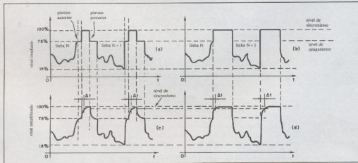
Fig. 11 - IV Comparação entre o padrão FCC e outro sem os pórtilcos de sincronismo, mostrando os respectivos sinais irradiados e amplificados.
