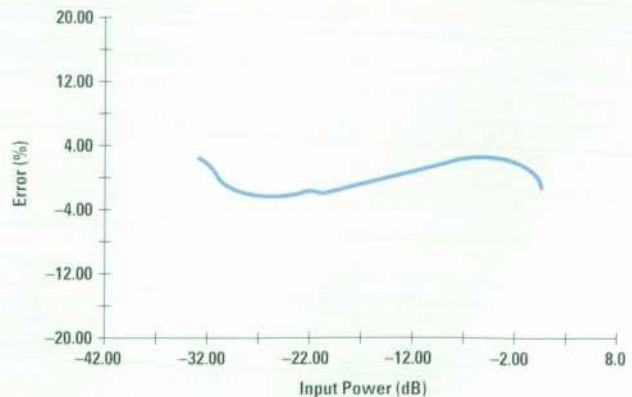
Fig. 20. Detector linearity error.
