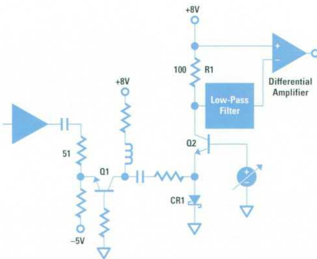
Fig. 18. Linear detector circuit.
