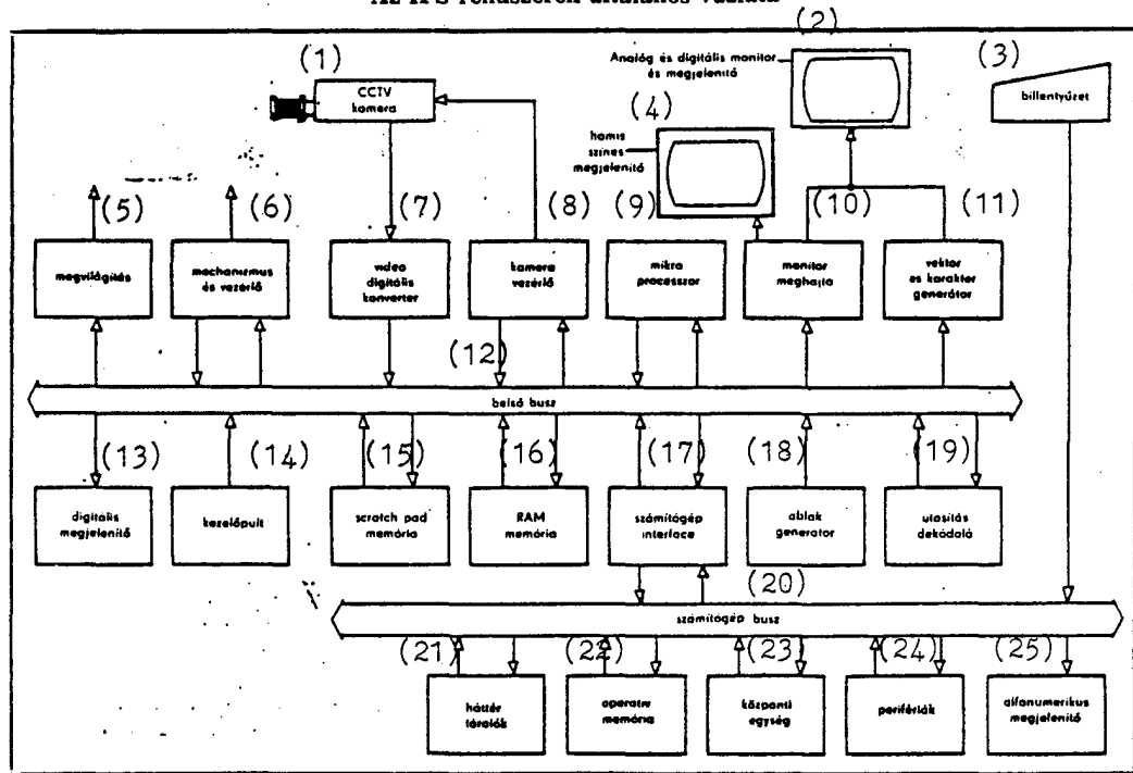
Az IPS rendszerek általános vázlata
