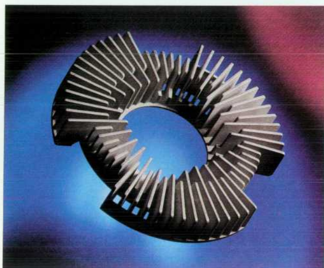
Fig. 4. Production part.
