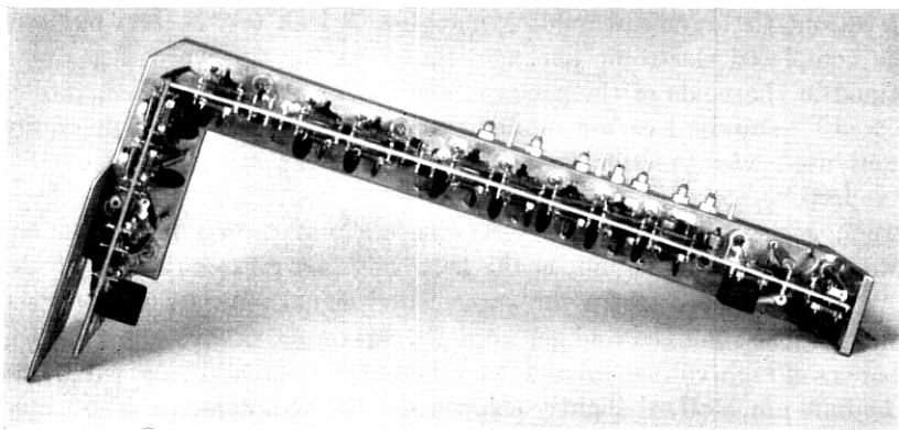
Fig. 16 — IF amplifier.
