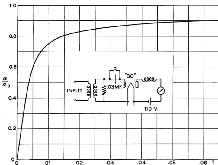
Fig. 12—Impulse meter.
