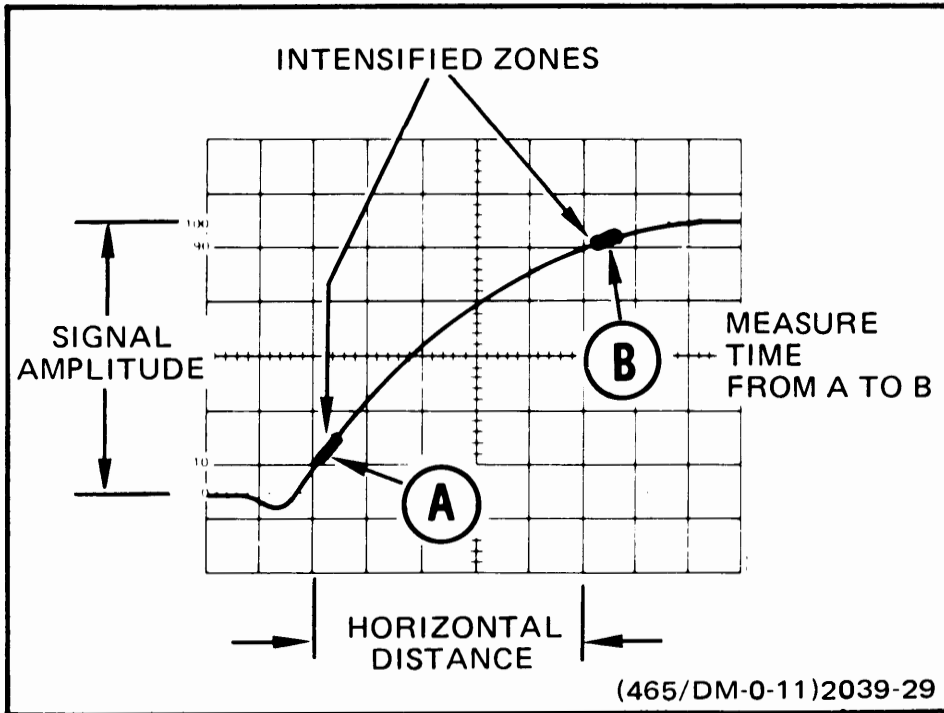
Fig. 28. Risetime.
