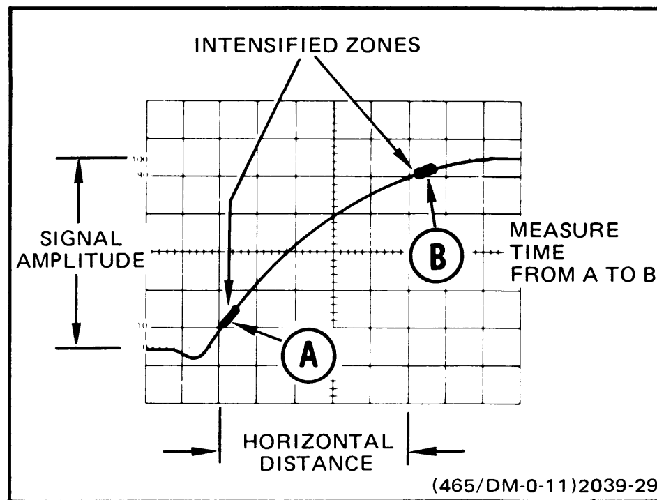
Fig. 32. Risetime.
