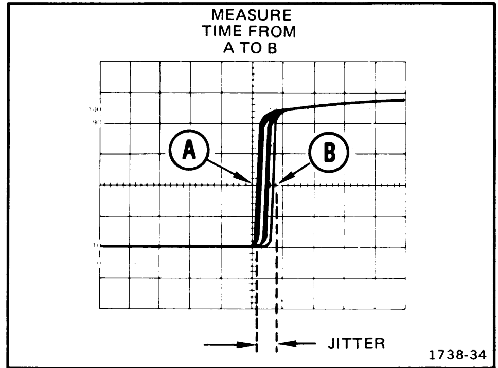
Fig. 23. Pulse jitter.
