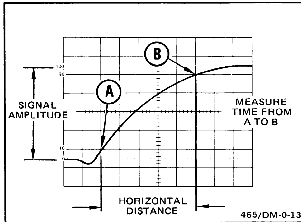
Fig. 19. Risetime.
