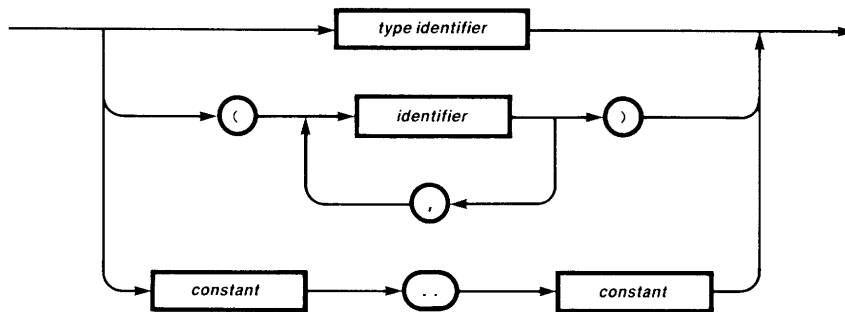
simple type
