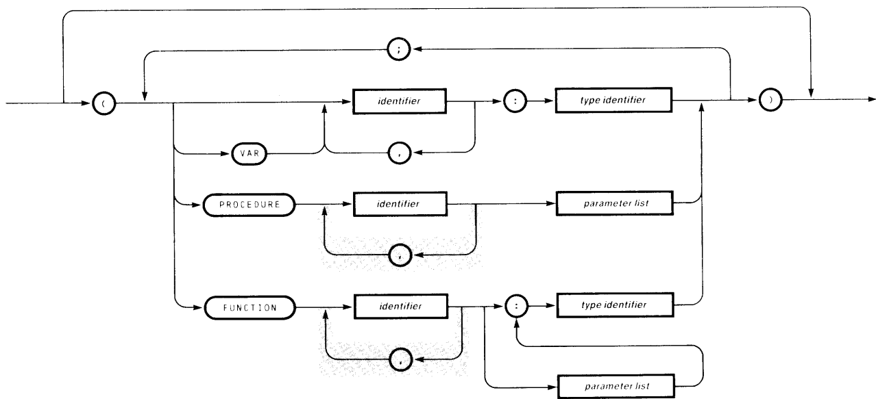
parameter list
